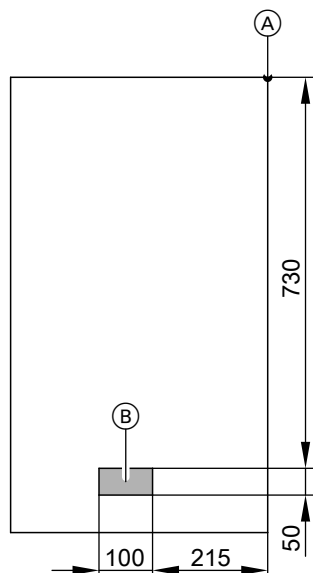
Vitodens 100-W
