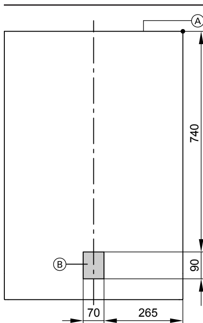
Vitodens 111-W
